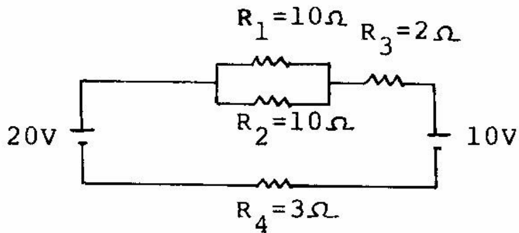
Circuito Pregunta 5878
