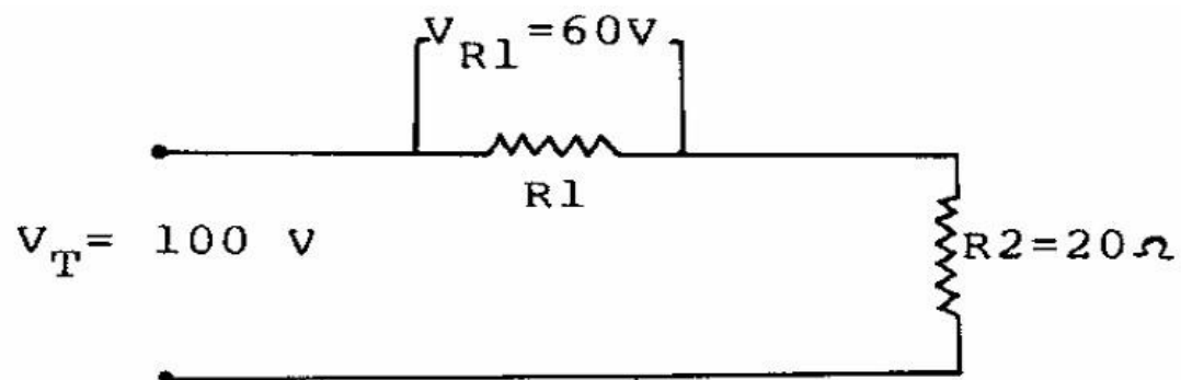
Circuito Pregunta 5049
