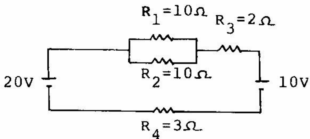
Circuito Pregunta 5096
